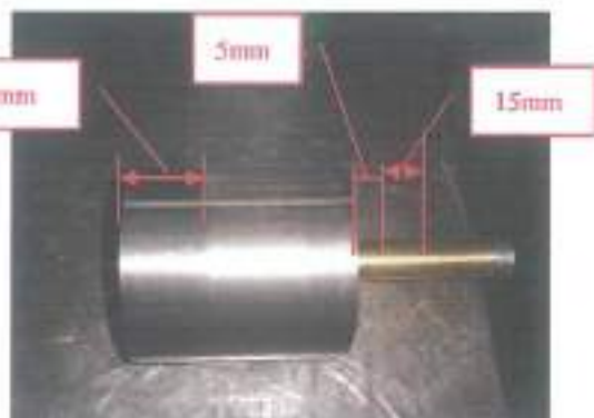
图 12 柱塞润滑脂涂抹位置
